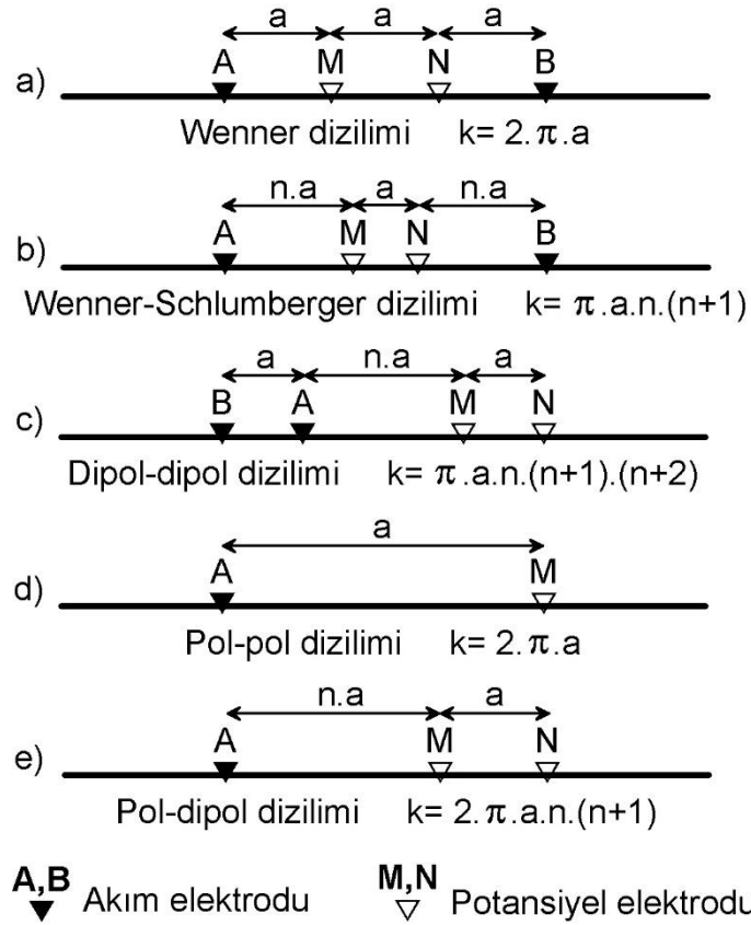
Şekil 3.1. a) Wenner, b) Wenner-Schlumberger, c) dipol-dipol, d) pol-pol ve e) pol-dipol dizimlerinde kullanılan elektrotların yüzeydeki dağılımı ve dizimlere ait geometrik faktör (k) hesabı.
